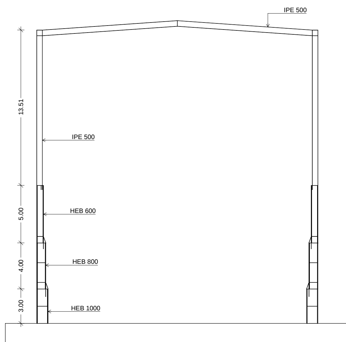
Pòrtic interior Escala 1:200
