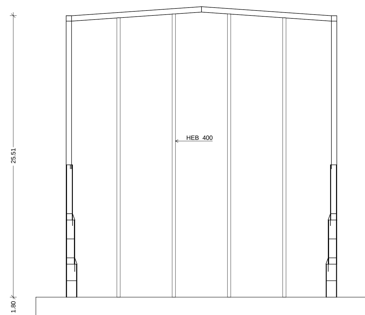
Pòrtic hastial Escala 1:200
